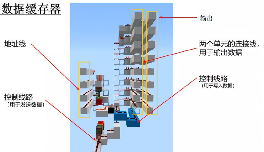
设计数据缓存器
